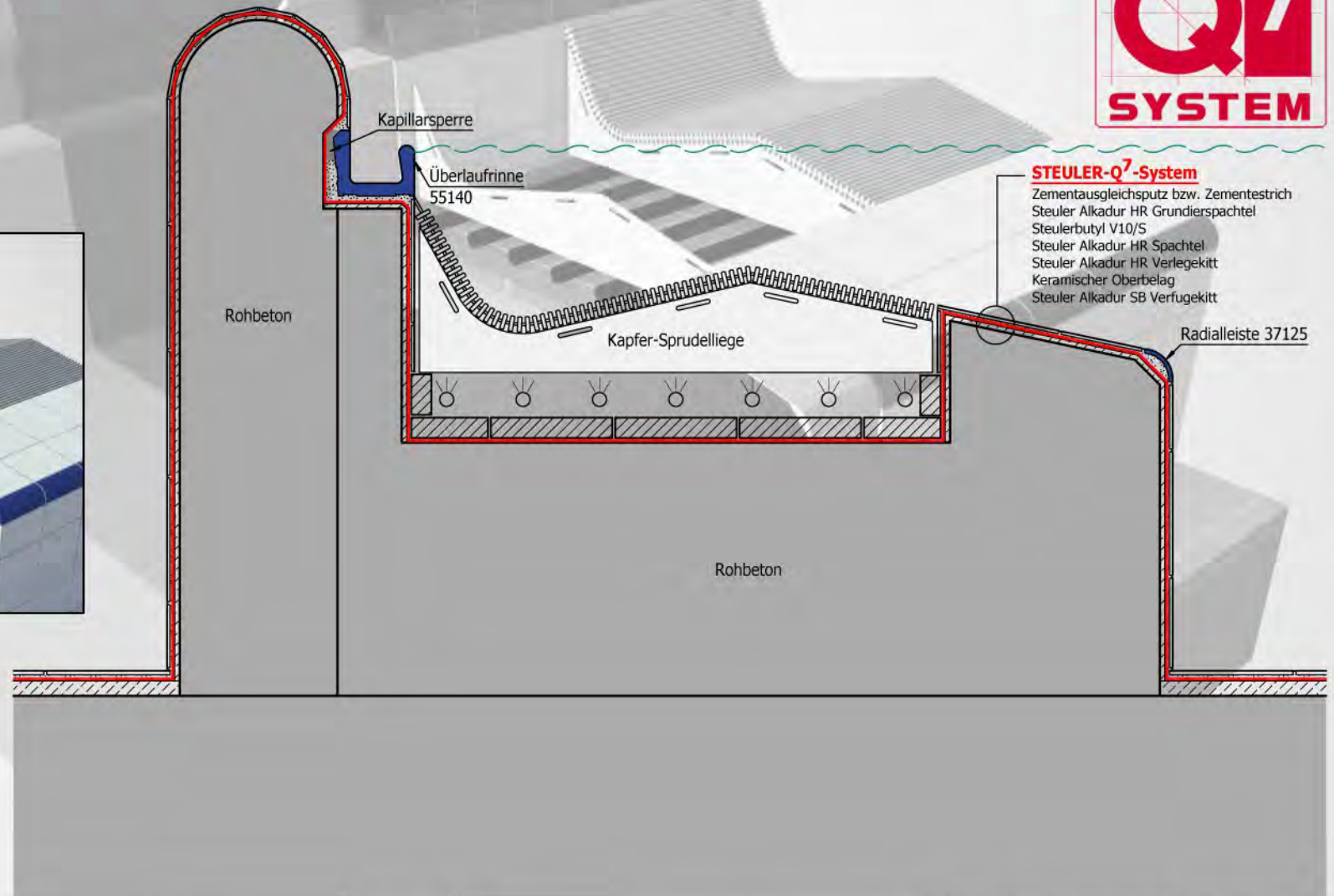
Systemschnitt 9.3 Sprudelliege
