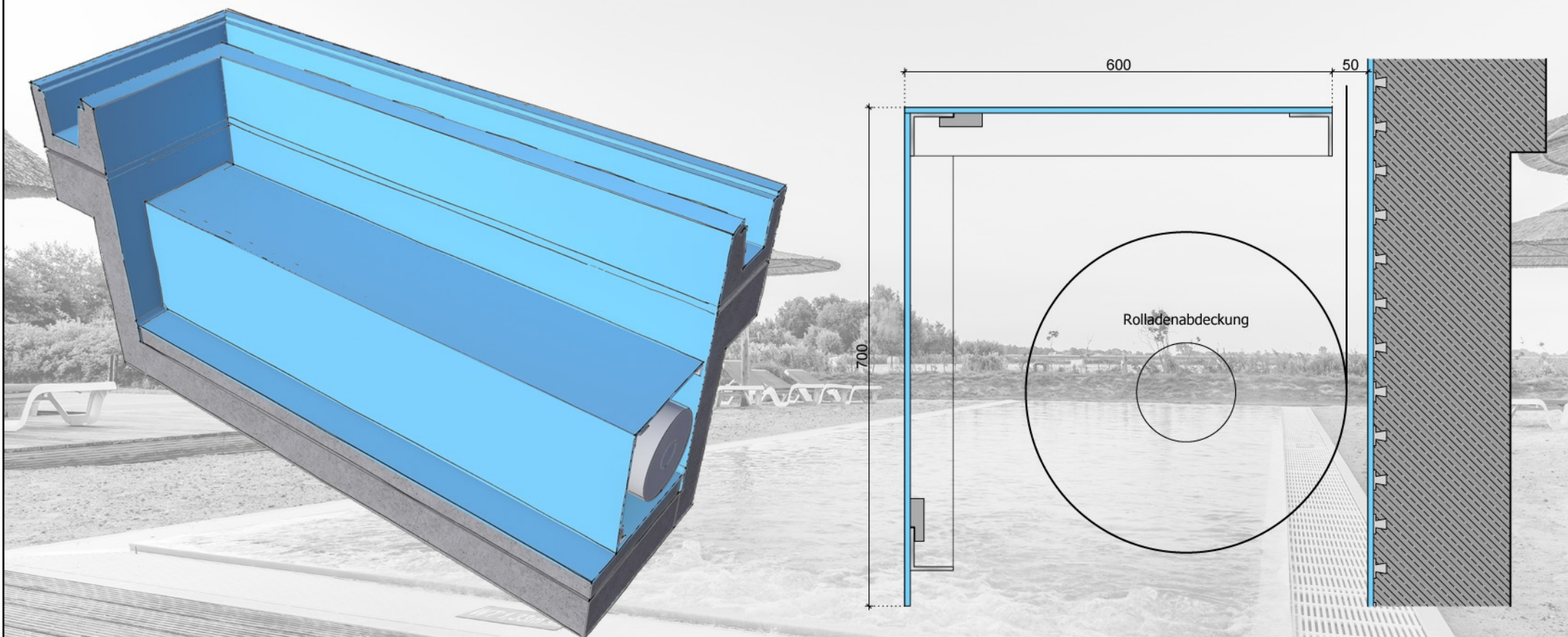
Systemschnitt 5.4 Sitzbank mit integriertem Rolladen
