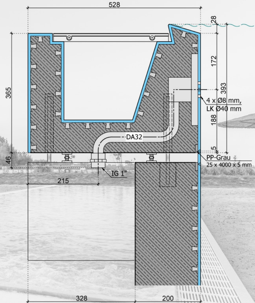
Systemschnitt 3.6 Rinnenelement mit Messwasserstutzen Anschluss nach unten
