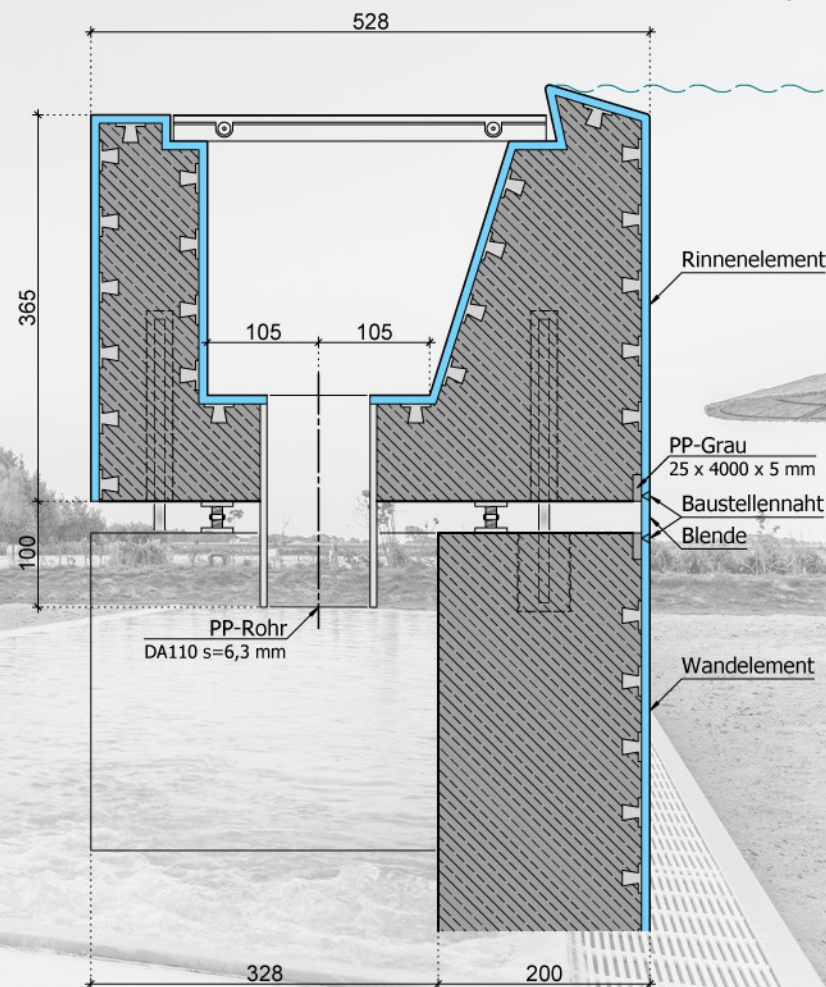
Systemschnitt 3.4 Rinnenelement mit Ablauf Anschluss über Rohrende
