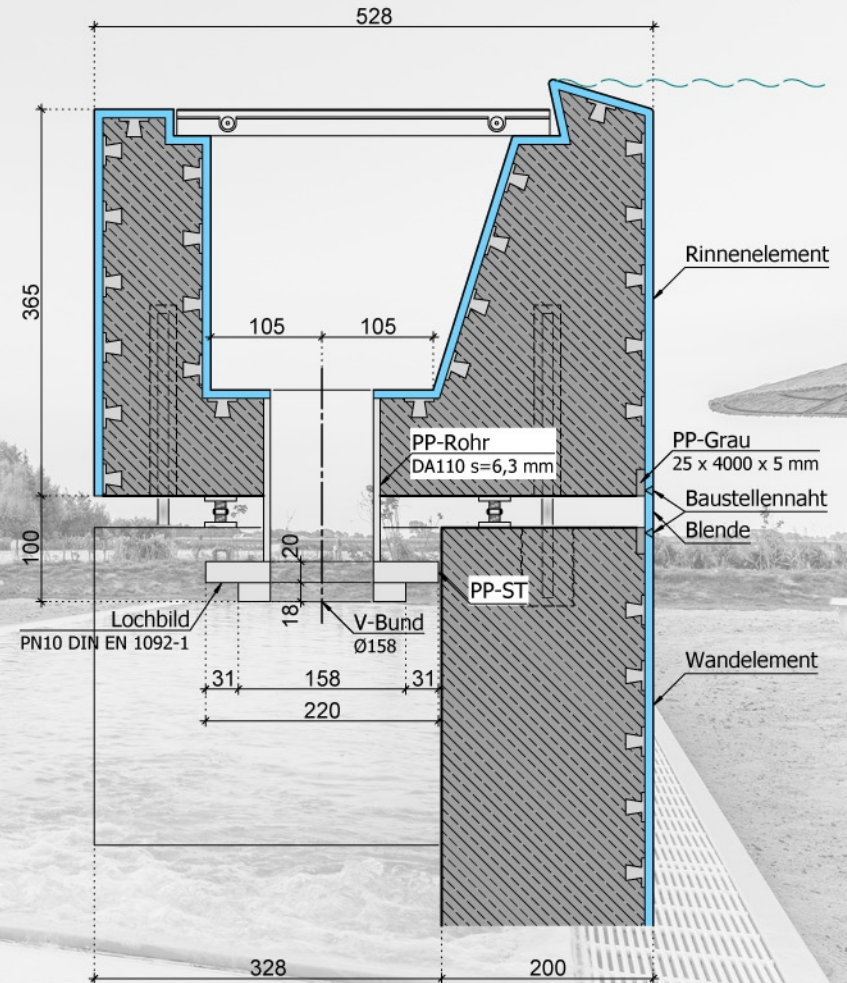
Systemschnitt 3.3 Rinnenelement mit Ablauf Anschluss über Flansch
