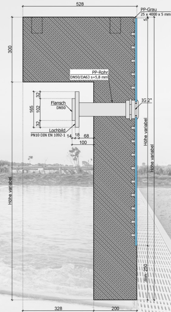
Systemschnitt 2.4 Wandelement mit Einströmdüse Anschluss über Flansch
