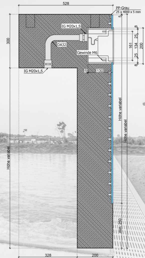
Systemschnitt 2.3 Wandelement mit UWS Anschluss nach unten
