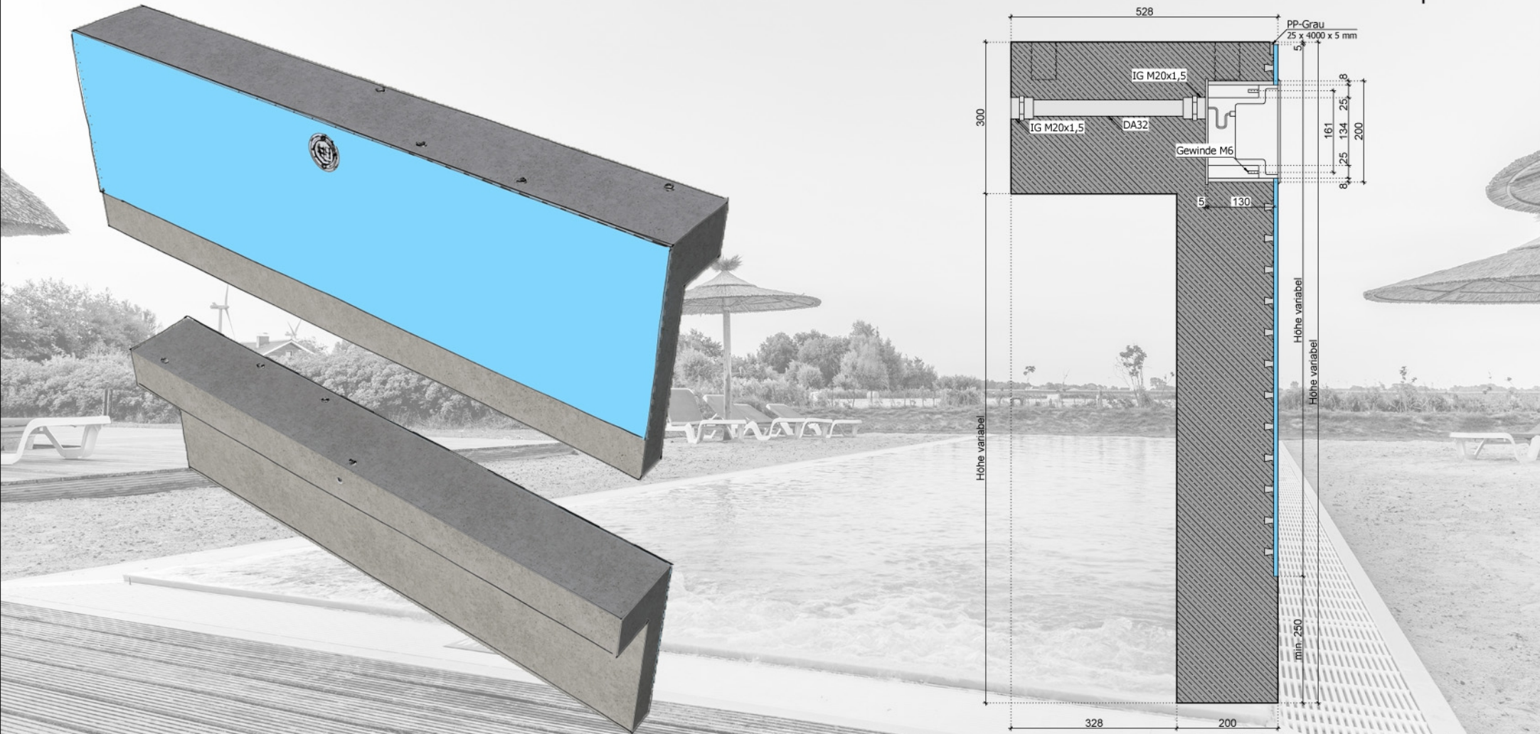
Systemschnitt 2.2 Wandelement mit UWS Anschluss nach hinten
